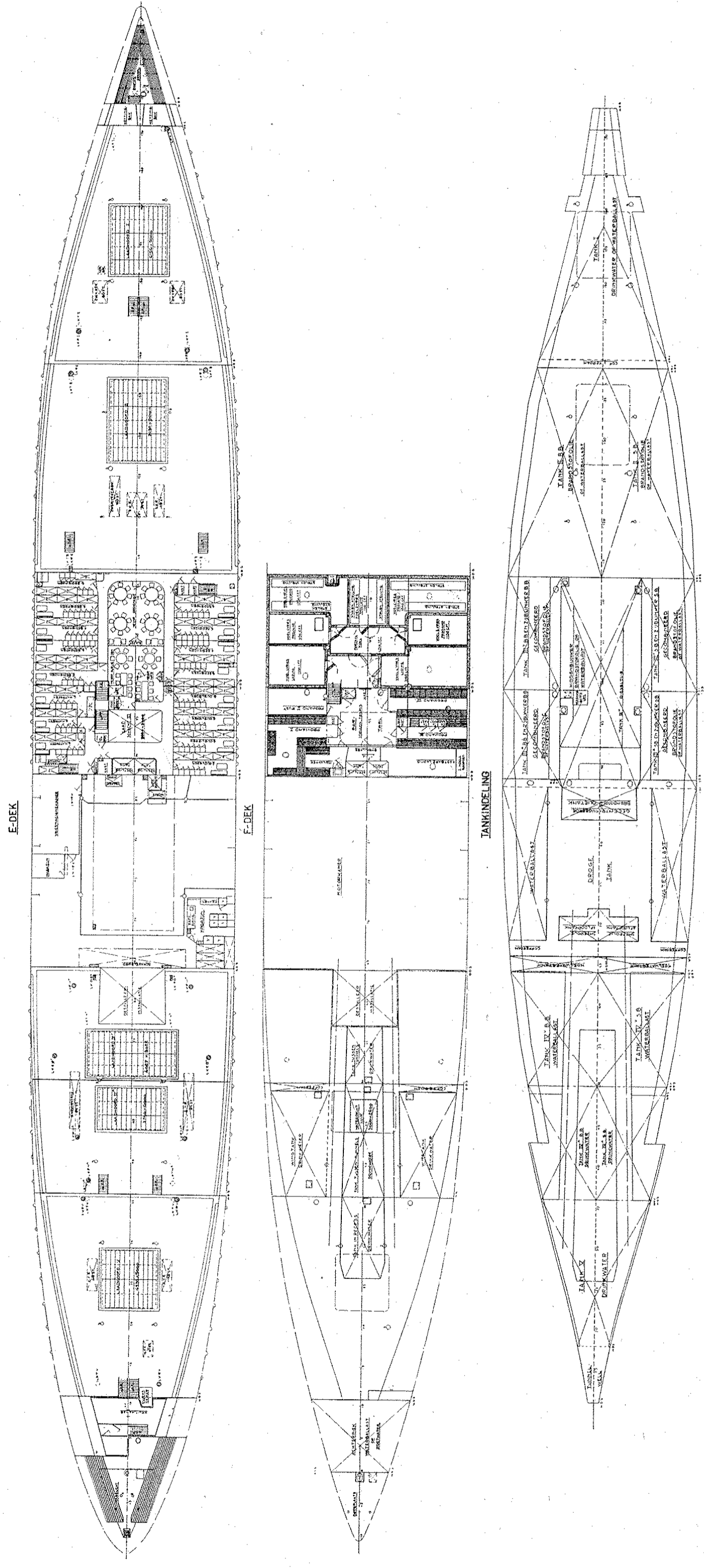
DEKENPLAN M.S. „TJIWANGI“, E-DEK, F-DEK, TANKINGDEK
