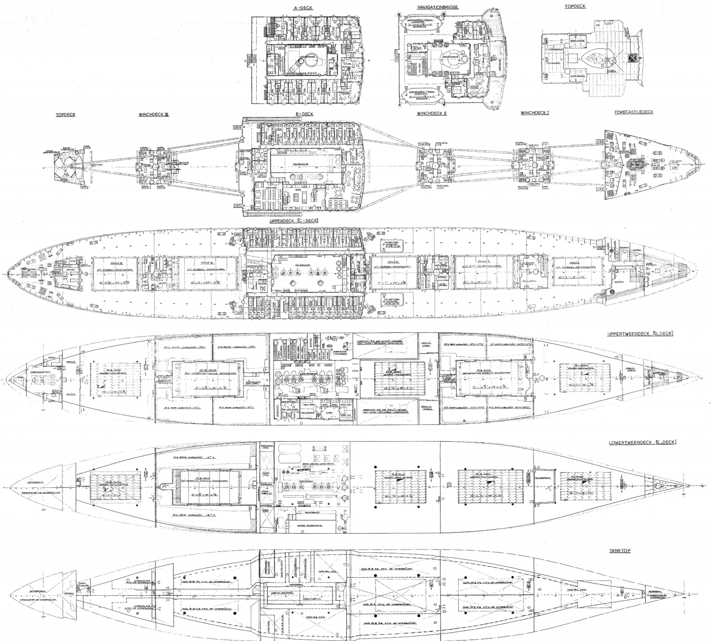
Algemeen plan m.s. „Straat Frazer” gebouwd door de Machinefabriek en Scheepswerf van P. Smit Jr., Rotterdam, bestemd voor de N.V. Koninklijke Paketvaart Maatschappij, Amsterdam. Afm.: lengte over alles 156,73 m; lengte tussen l.l. 142,25 m; breedte op spanten 20,42 m; holte tot bovenste dek 12,192 m; diepgang (zomer) 9,45 m; draagvermogen hierbij 12.284 ton; bruto tonnage 9.294 r.t.; netto tonnage 5.177 r.t.
