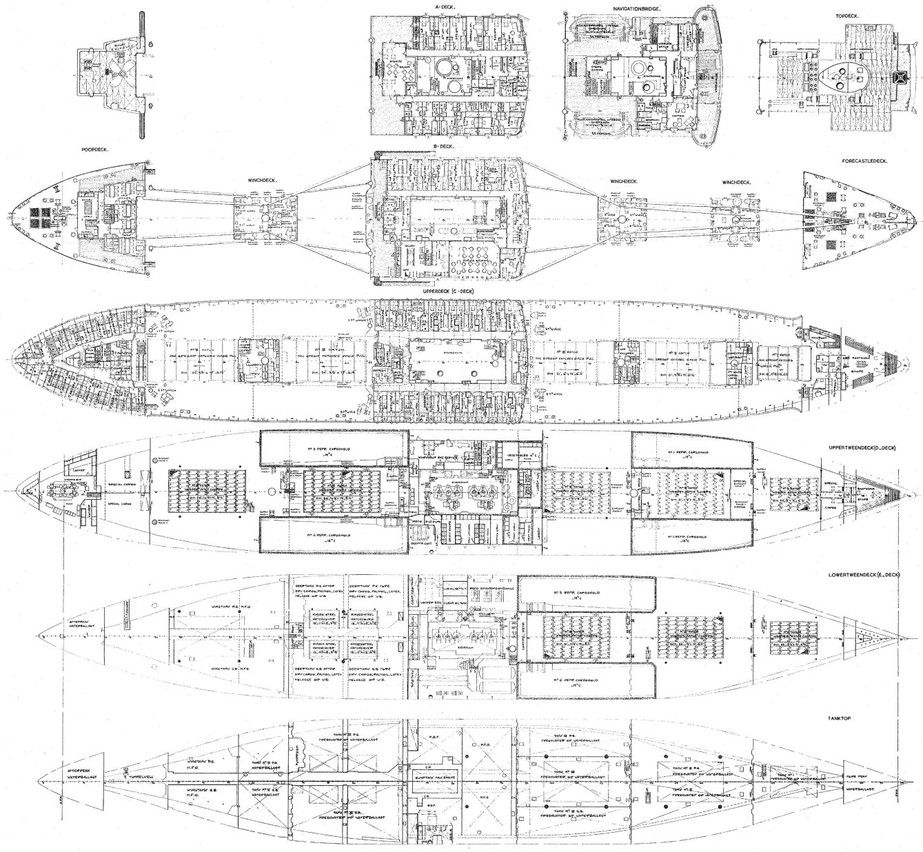
ALGEMEEN PLAN EN DEKKENPLAN M.S. „STRAAT CLARENCE“
