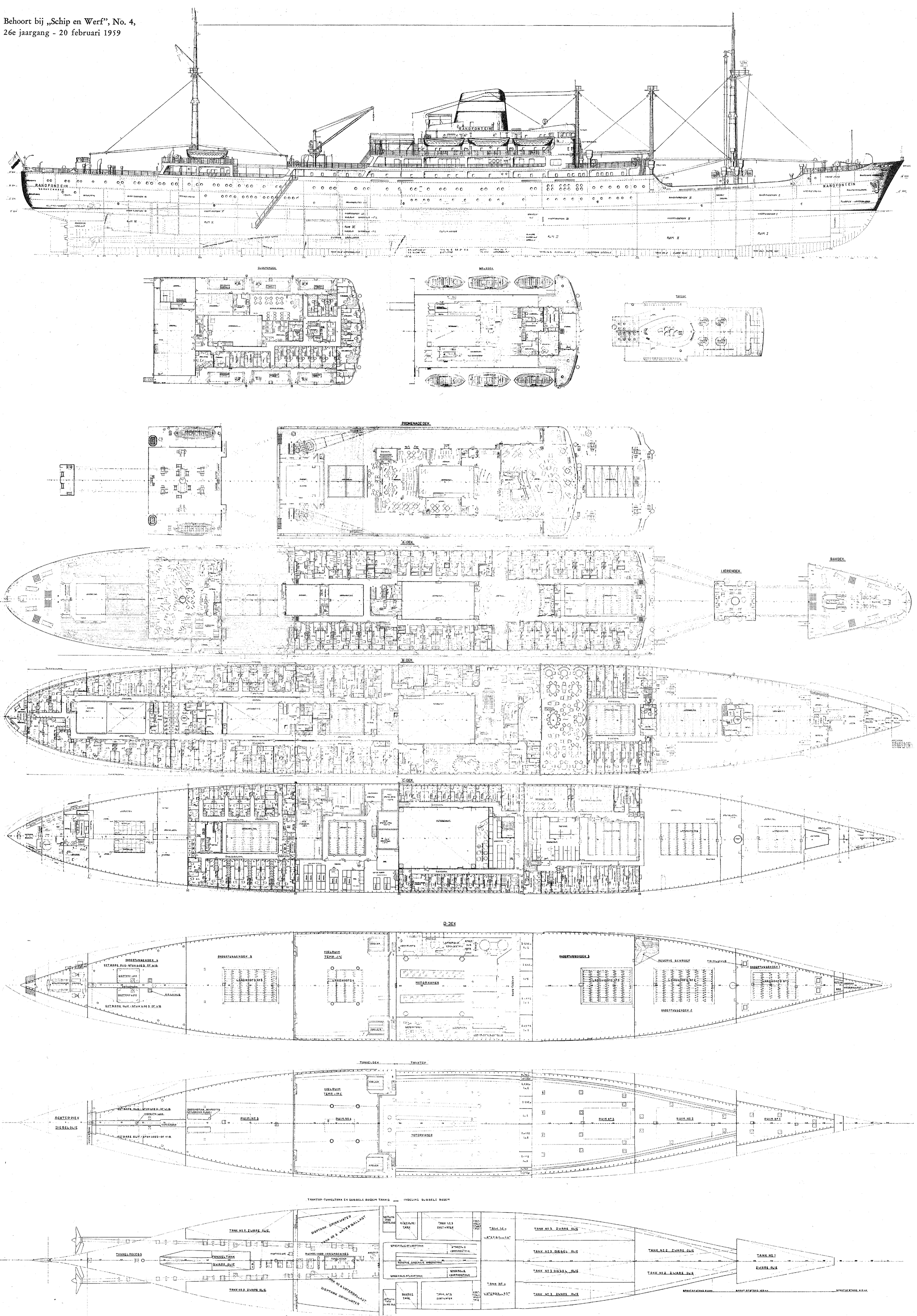
Dubbelschroefmotor passagiersschip „Randfontein” Algemeen plan en dekkenplan
